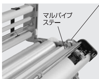
第6図 スリッターフックをかけます。
