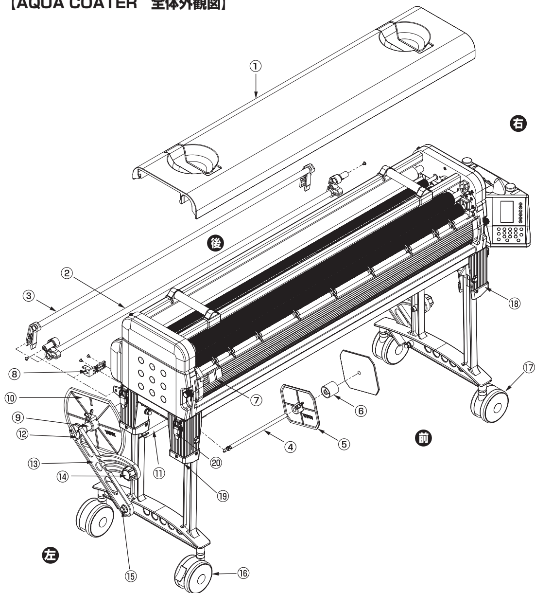
【全体外観図】
