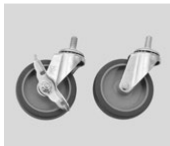
409-840 φ100mmキャスターF(ストッパー有) 409-841 φ100mmキャスターF(ストッパー無) ※薄型スパナ(19×21mm)を使用し、交換できます。
