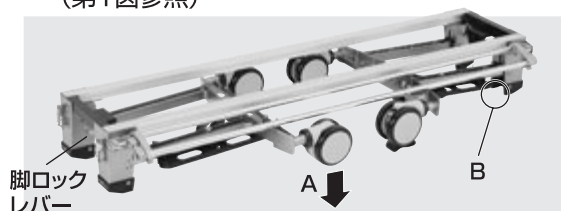
第1図(脚部を折りたたんだ状態)
