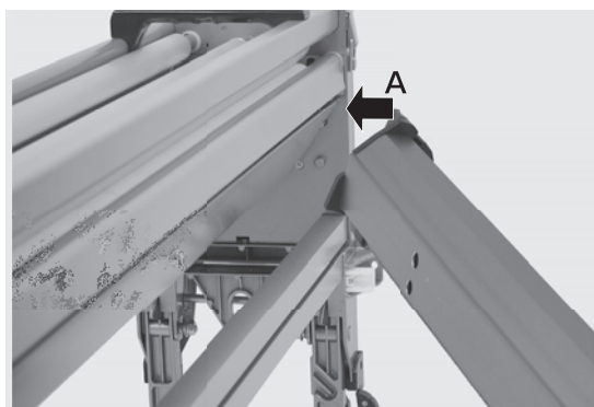
第7図（スリッターを引っかけた状態）
