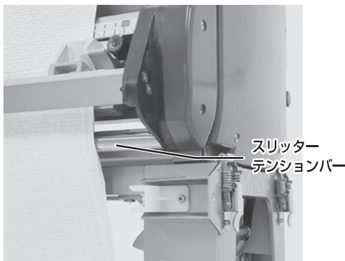
第19図(スリッターテンションバー解除状態)
